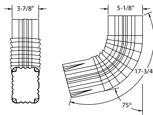
ABE245 B-Elbow
