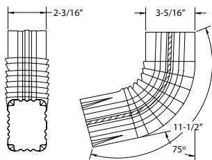
AAE245 A-Elbow
