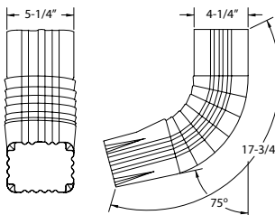
AAE245 A-Elbow
